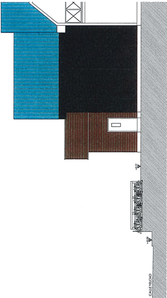
ELEVACIÓN PONIENTE SUM SITUACIÓN PROPUESTA ESCALA 1:50
