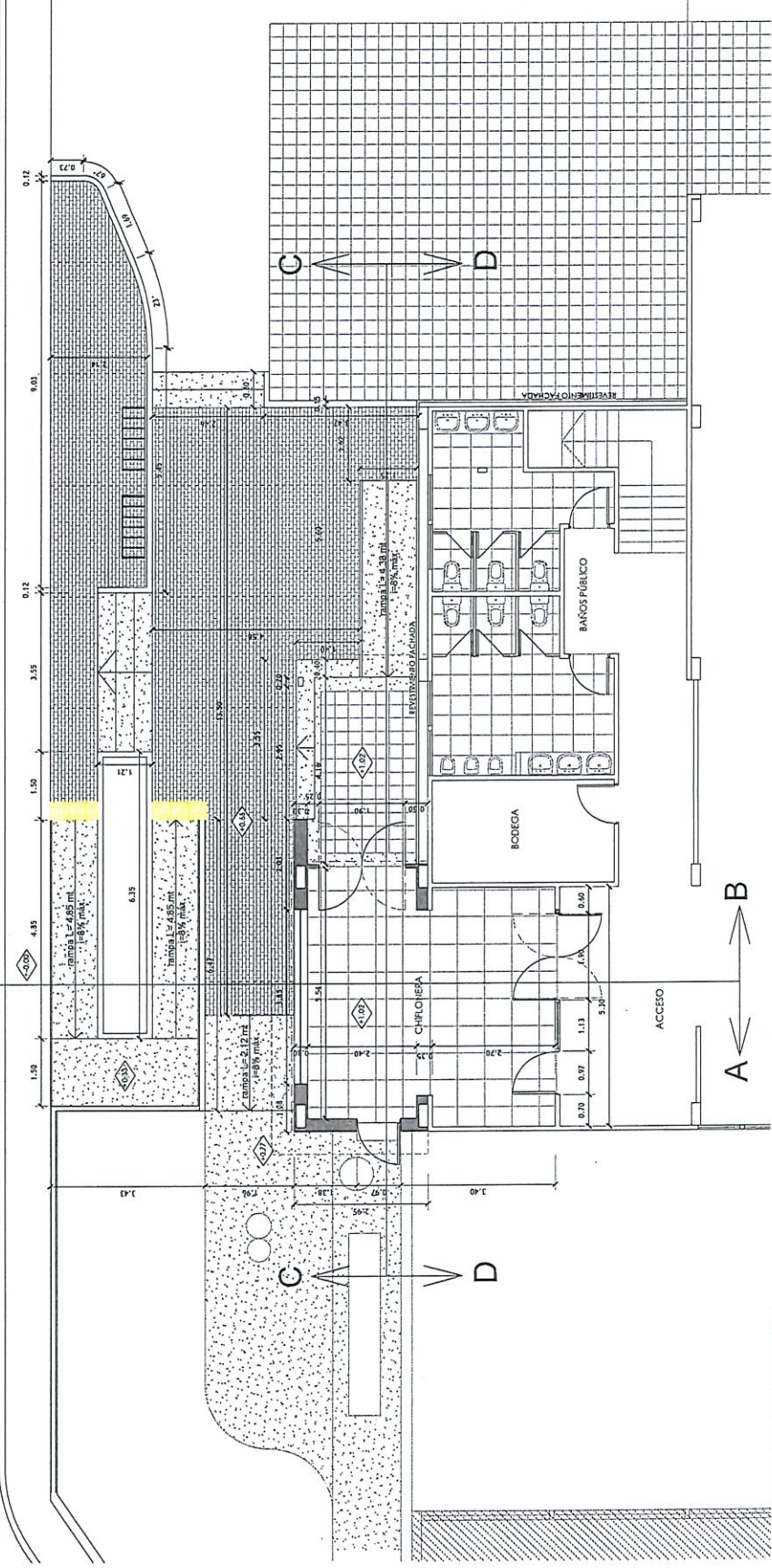
PLANTA SECTOR ACCESO SUM SITUACIÓN PROPUESTA ESCALA 1:50
