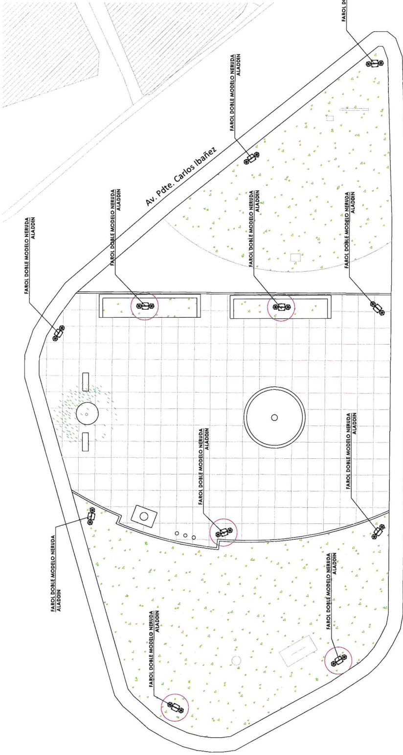
PLANTA UBICACIÓN FAROLES PROPUESTOS ESCALA 1:50
